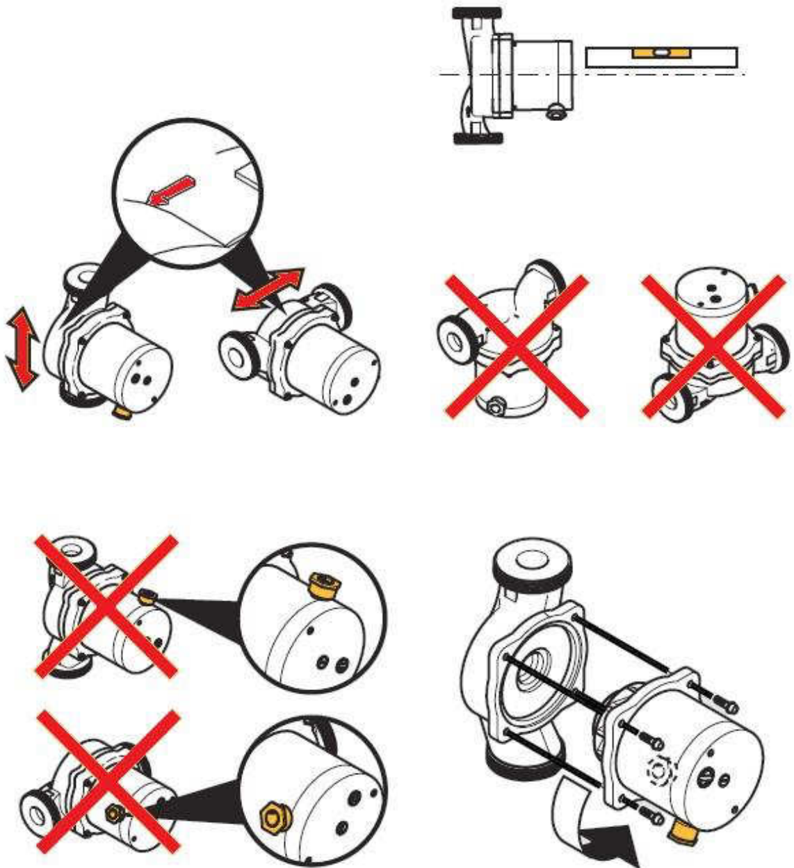
Bild: Pumpeneinbau
