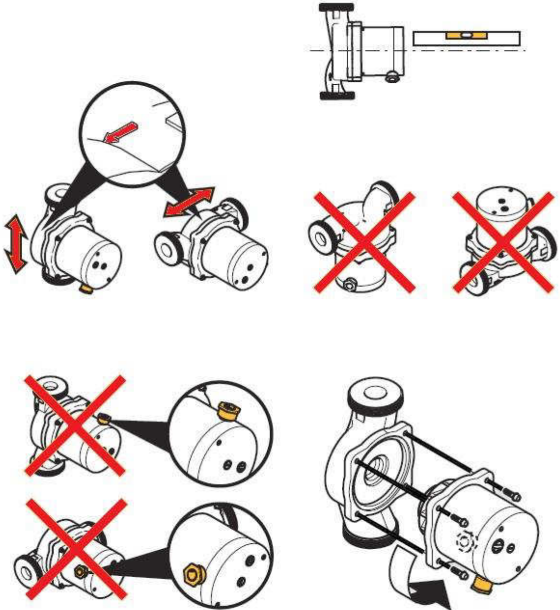
Bild: Pumpeneinbau
